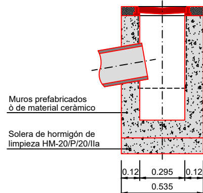
SECCIÓN A-A'
