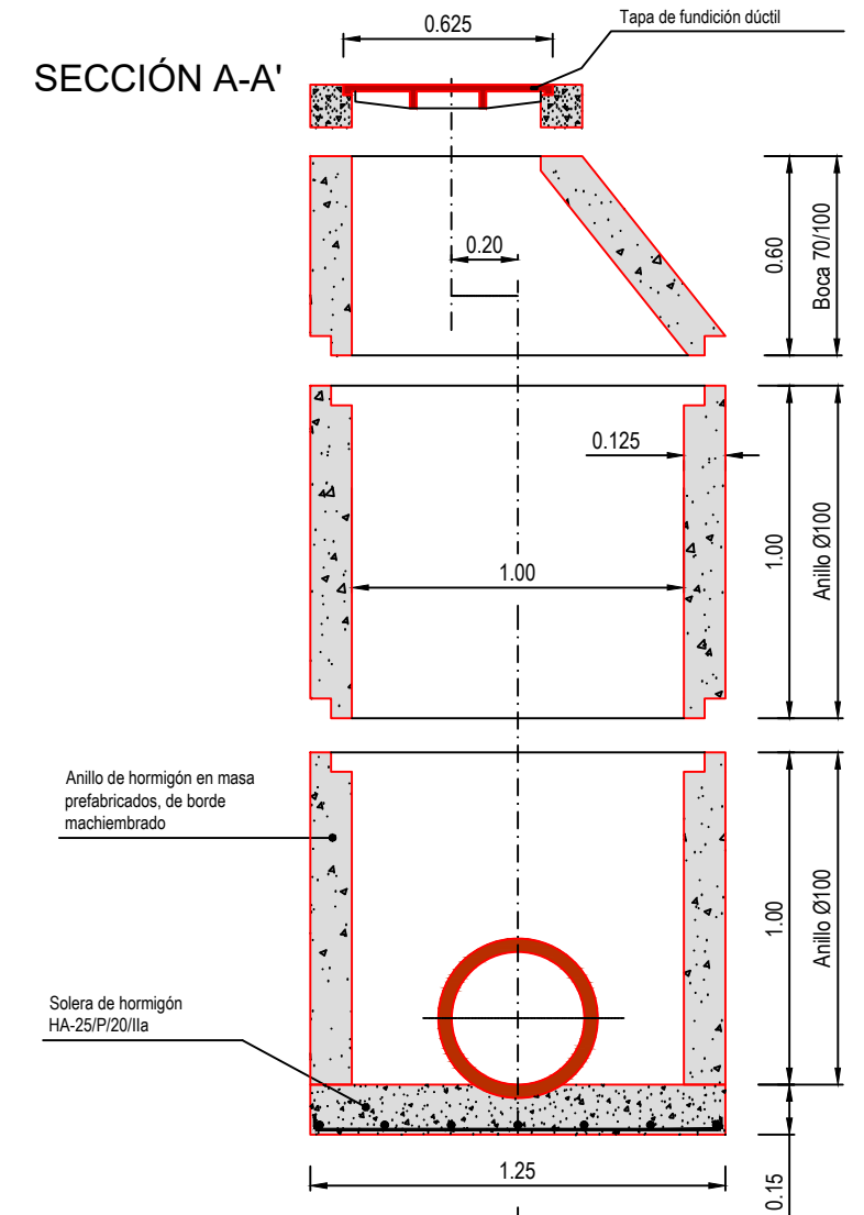
PLANTA-SECCION
