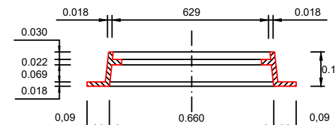
PLANTA-SECCION
